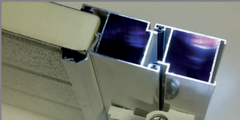
Konstrukční schéma horizontálních vrat ALU WD s nepřerušným tepelným mostem.
